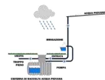
SCHEMA RECUPERO ACQUE PIOVANE
